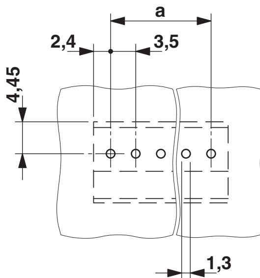
boorsjabloon/soldeerpadgeometrie
