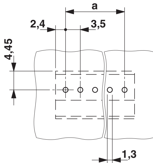
boorsjabloon/soldeerpadgeometrie
