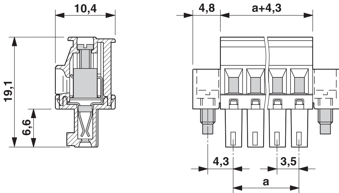
Maatschets
