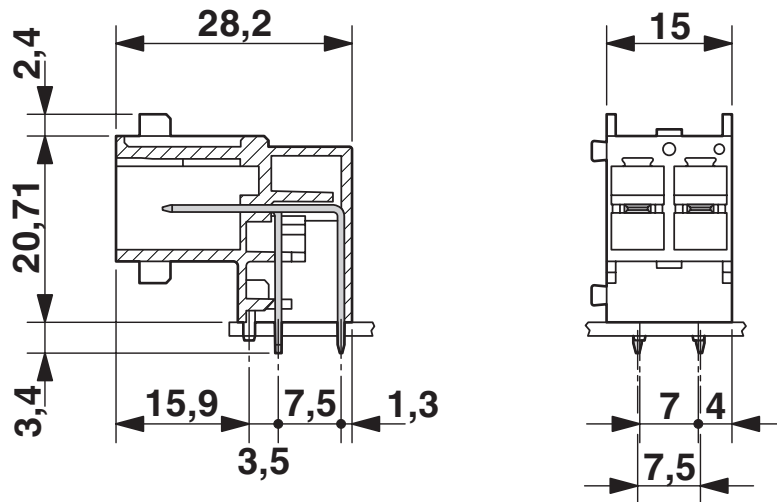
Maatschets
