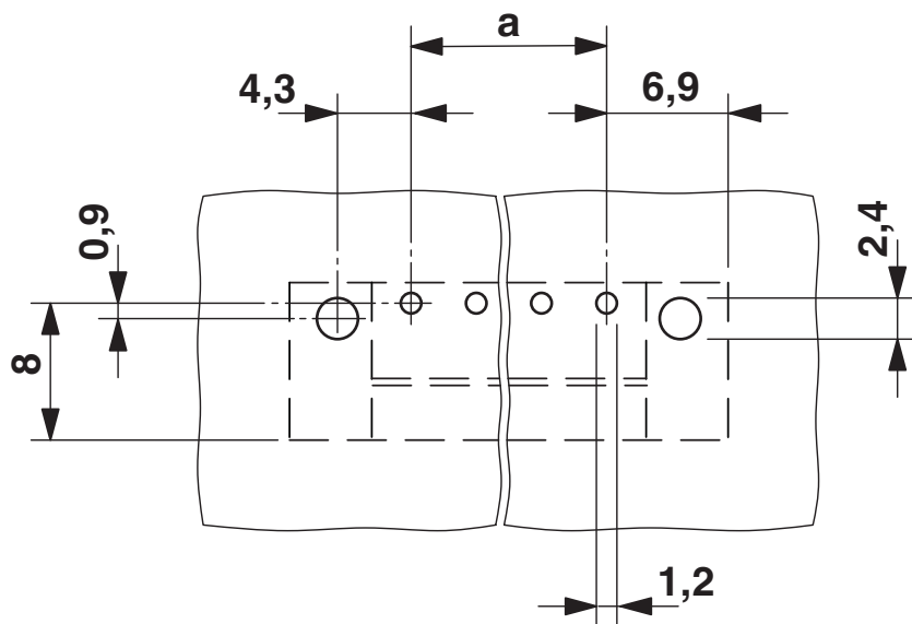
boorsjabloon/soldeerpadgeometrie
