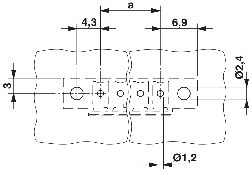
boorsjabloon/soldeerpadgeometrie
