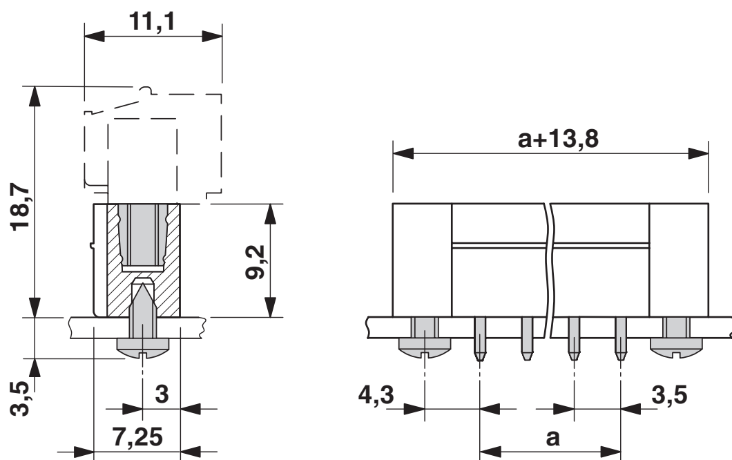
Maatschets
