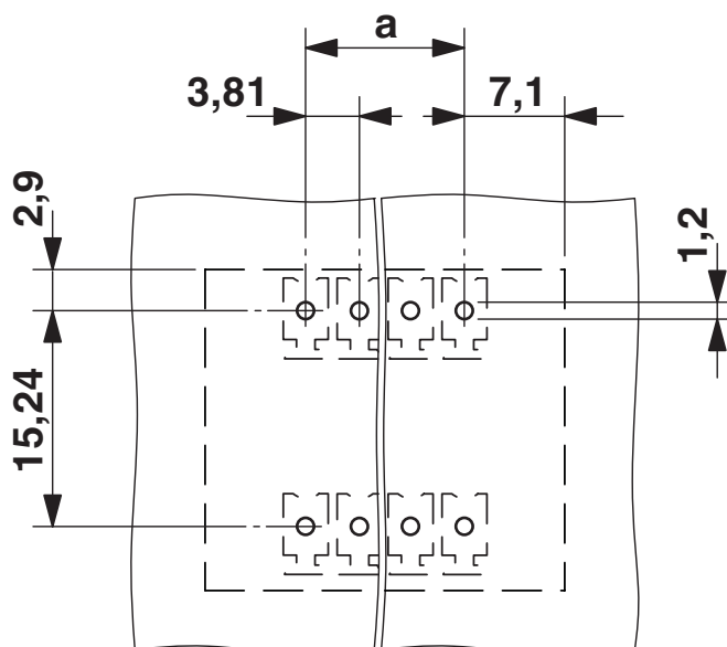
boorsjabloon/soldeerpadgeometrie
