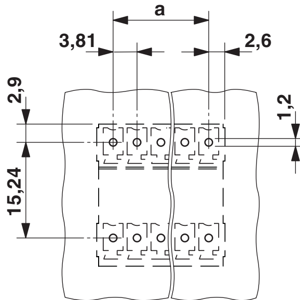
boorsjabloon/soldeerpadgeometrie
