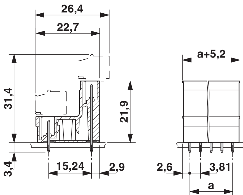
Maatschets
