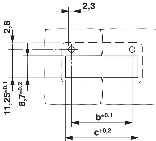
boorsjabloon/soldeerpadgeometrie
