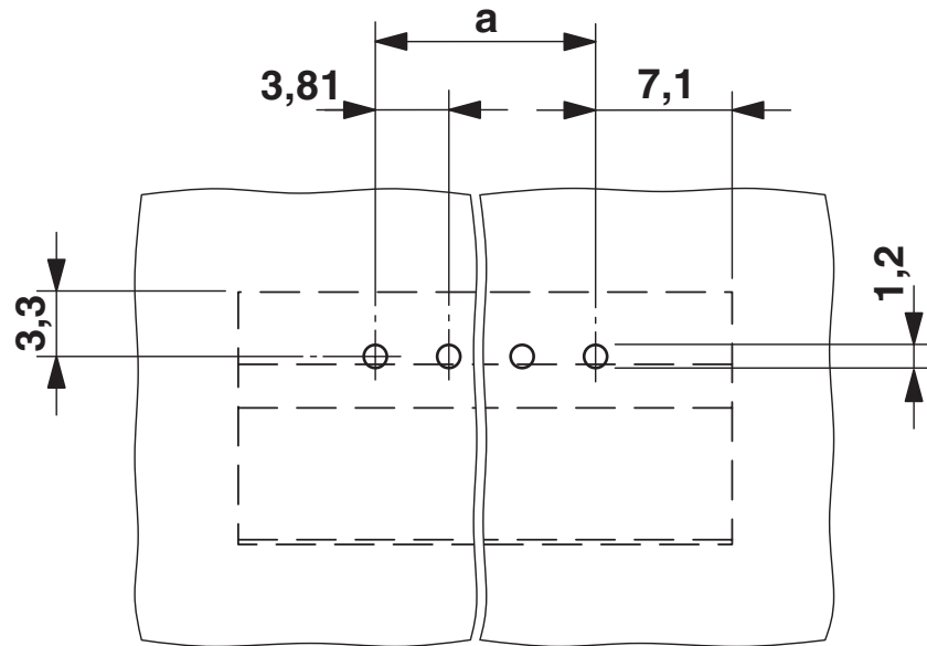
boorsjabloon/soldeerpadgeometrie
