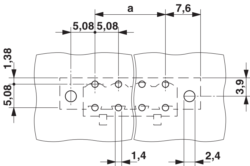
boorsjabloon/soldeerpadgeometrie
