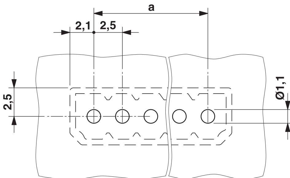
boorsjabloon/soldeerpadgeometrie
