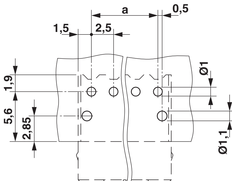
boorsjabloon/soldeerpadgeometrie
