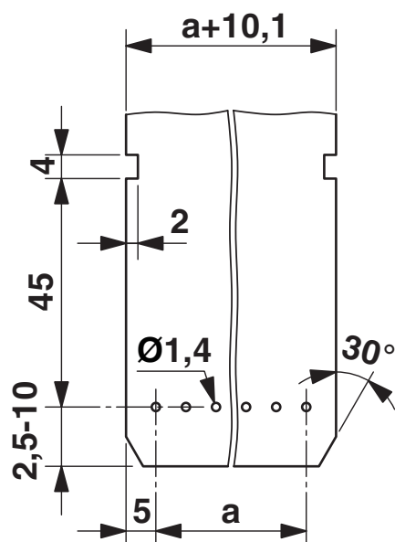
boorsjabloon/soldeerpadgeometrie
