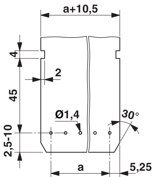
boorsjabloon/soldeerpadgeometrie
