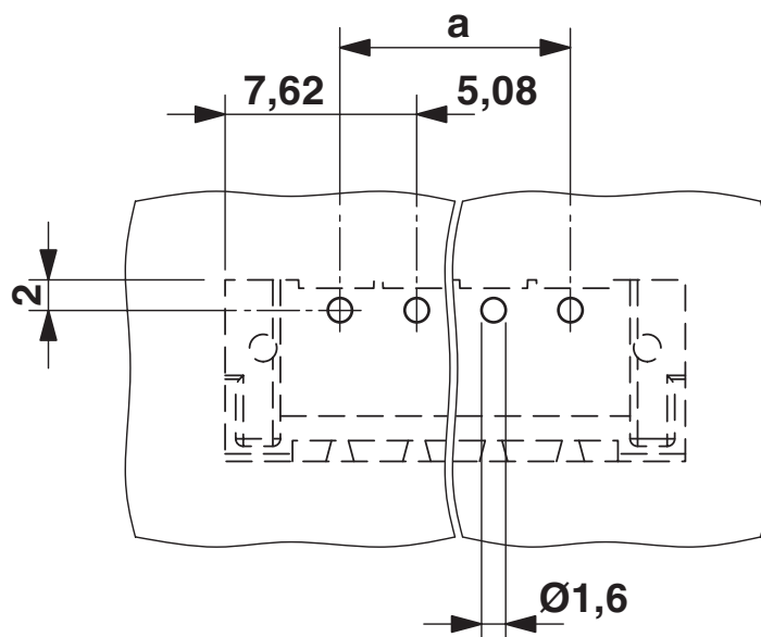
boorsjabloon/soldeerpadgeometrie
