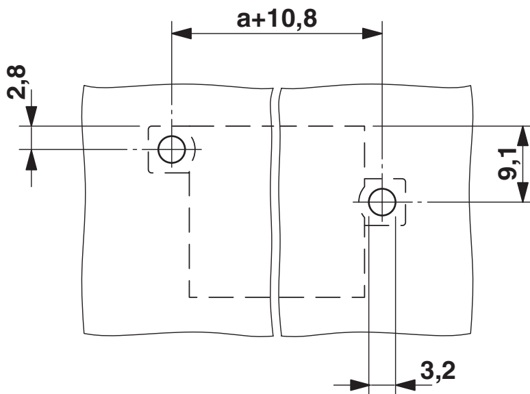
boorsjabloon/soldeerpadgeometrie
