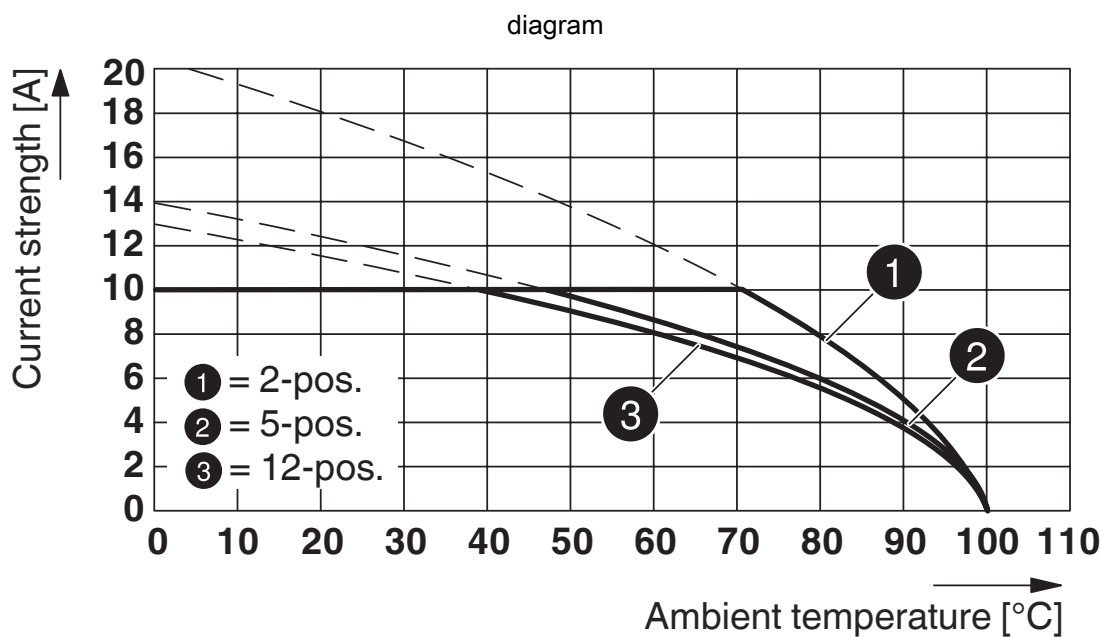
Type: MVSTB(R/W) 2,5/...-ST-5,08 met MDSTBW 2,5/...-G-5,08
