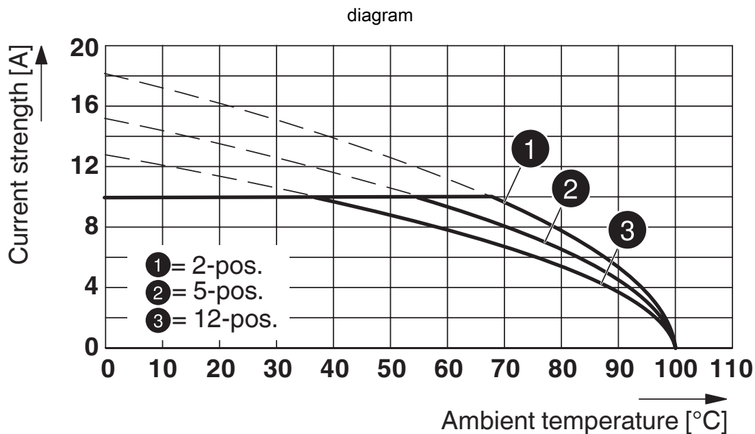
Type: MVSTBW 2,5/...-ST-5,08 met MDSTB 2,5/...-G-5,08
