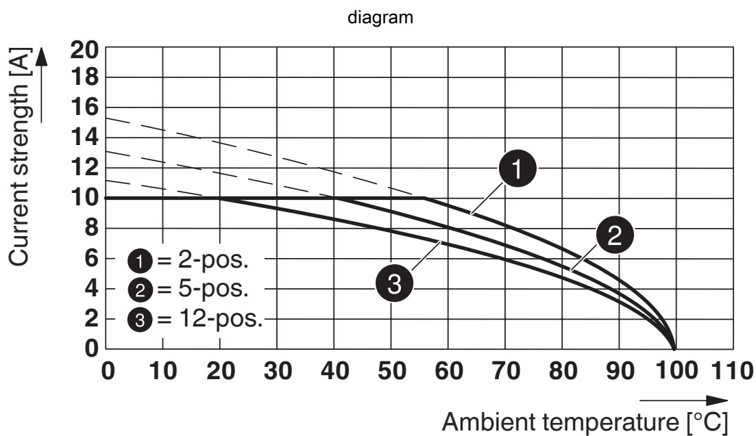
Type: MVSTB(R/W) 2,5/...-ST met MDSTBV 2,5/...-G-5,08
