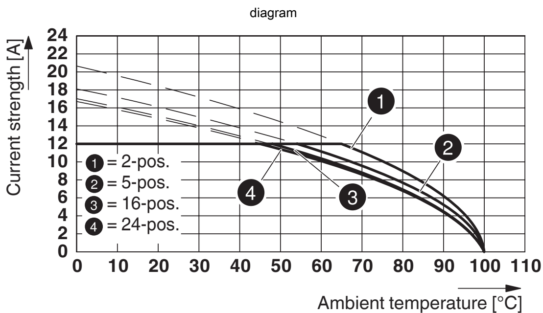
Type: MVSTBR 2,5/...-ST-5,08 met MSTBVK 2,5/...-G-5,08
