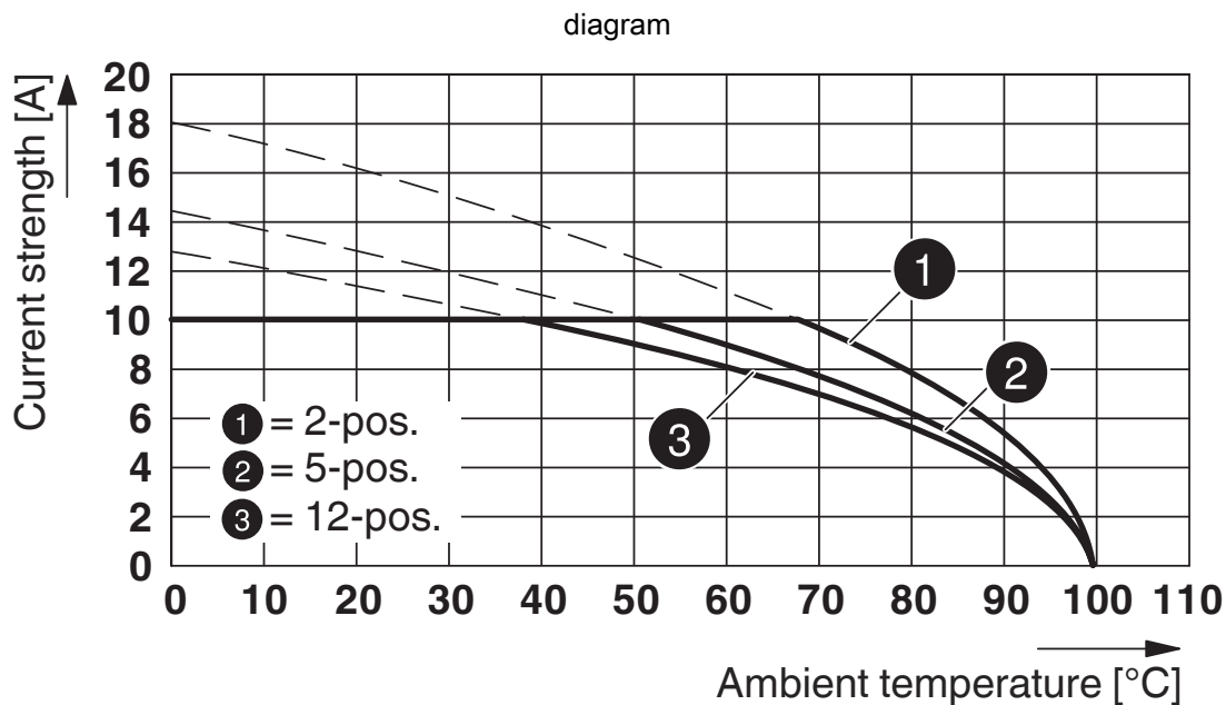
Type: MVSTB(R/W) 2,5/...-ST-5,08 met MDSTBA 2,5/...-G-5,08
