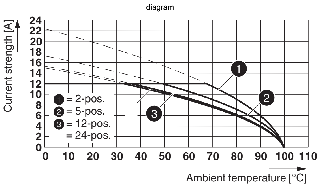
Type: MVSTB(R/W) 2,5/...-ST-5,08 met MSTB 2,5/...-G-5,08
