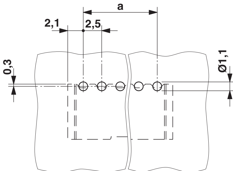
boorsjabloon/soldeerpadgeometrie
