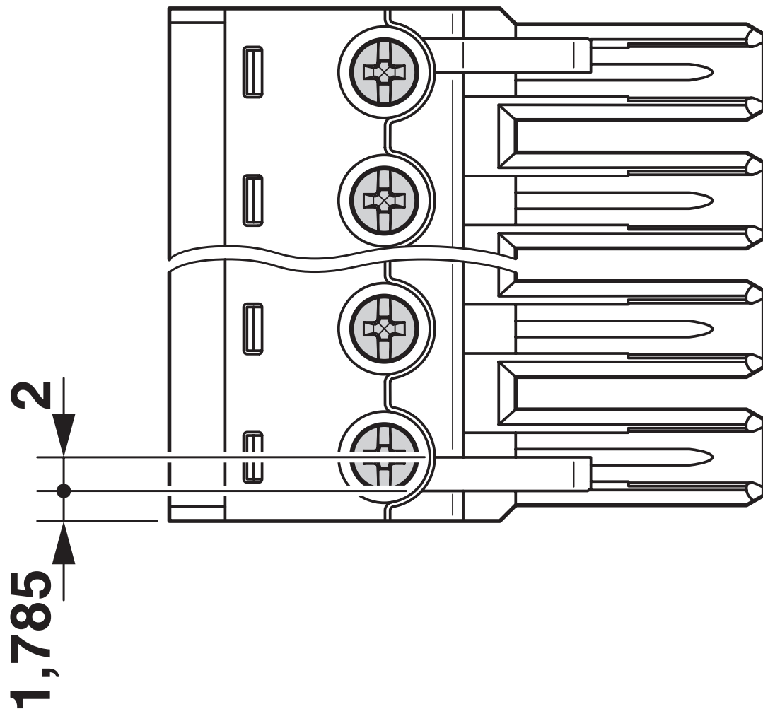
Maatschets
