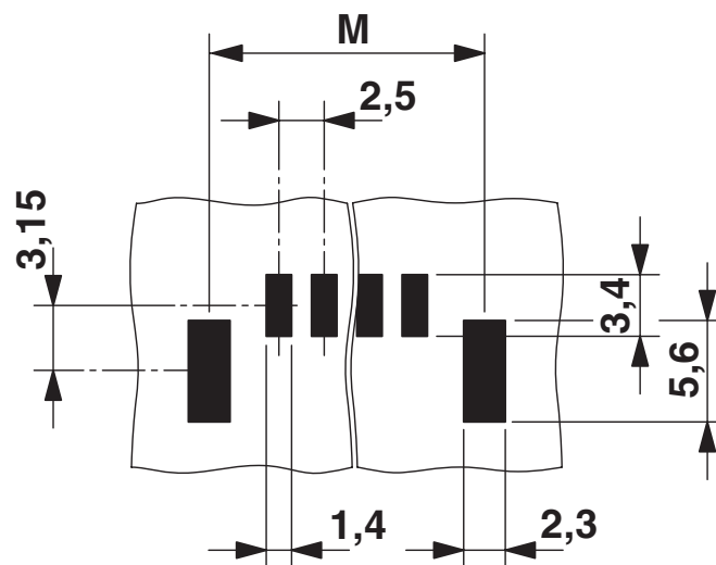
boorsjabloon/soldeerpadgeometrie
