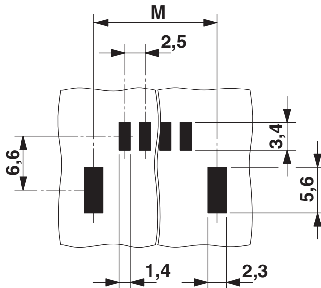
boorsjabloon/soldeerpadgeometrie
