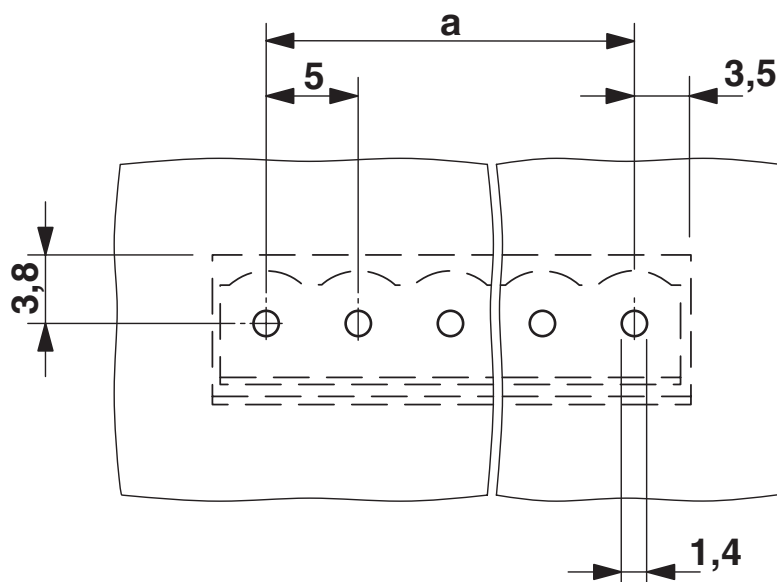
boorsjabloon/soldeerpadgeometrie
