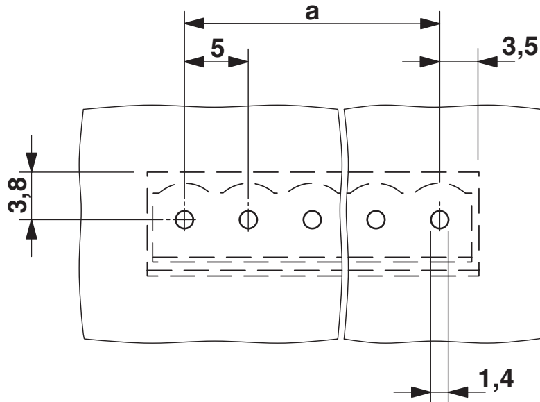
boorsjabloon/soldeerpadgeometrie
