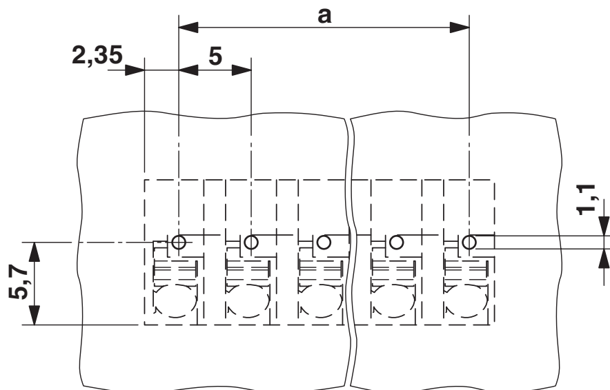
boorsjabloon/soldeerpadgeometrie
