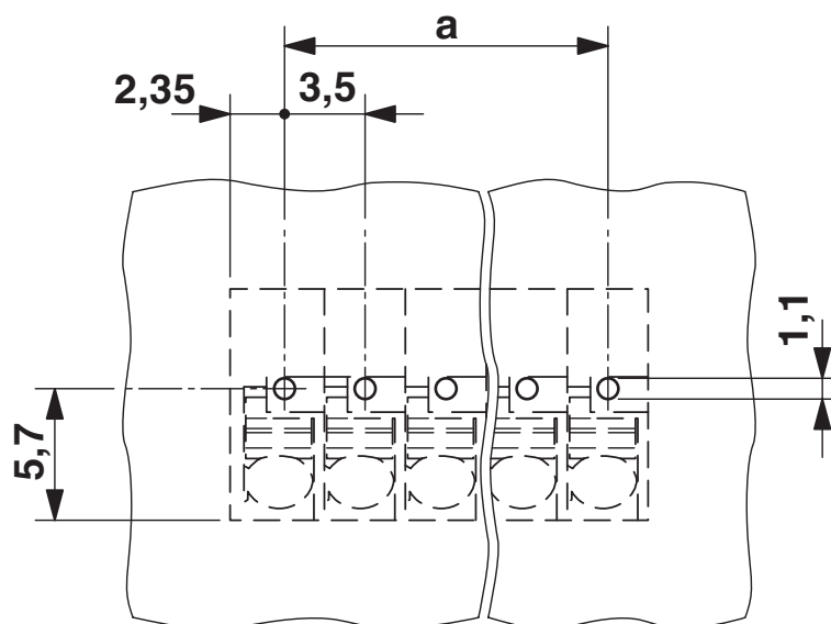
boorsjabloon/soldeerpadgeometrie
