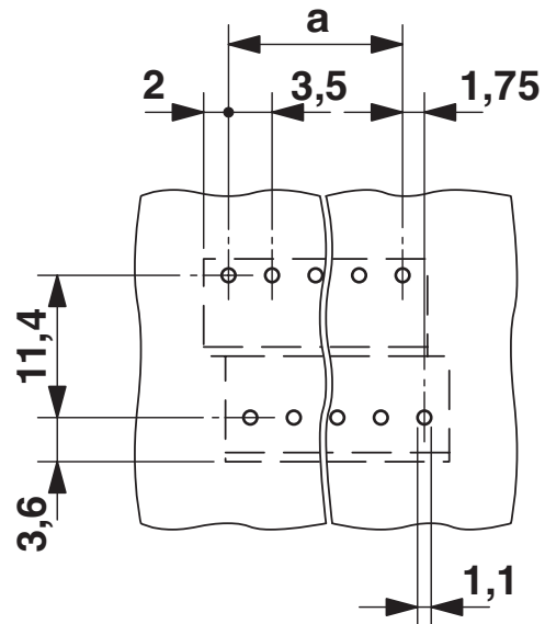
boorsjabloon/soldeerpadgeometrie
