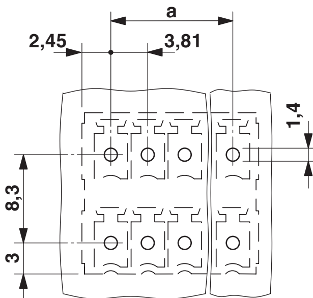
boorsjabloon/soldeerpadgeometrie
