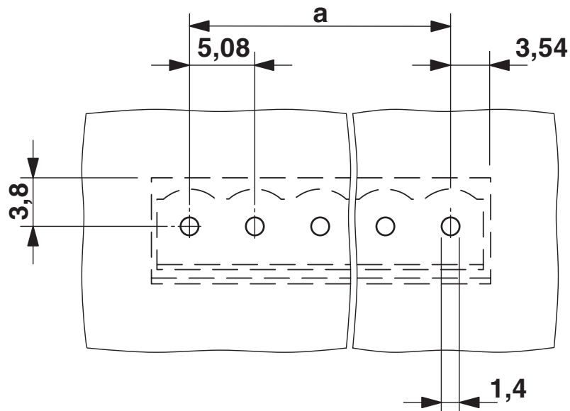
boorsjabloon/soldeerpadgeometrie
