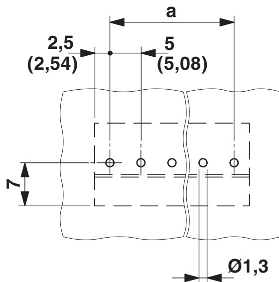
boorsjabloon/soldeerpadgeometrie
