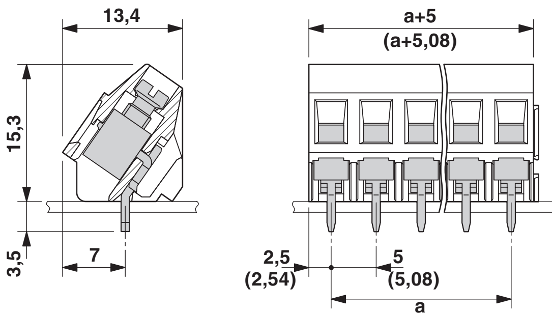
Maatschets
