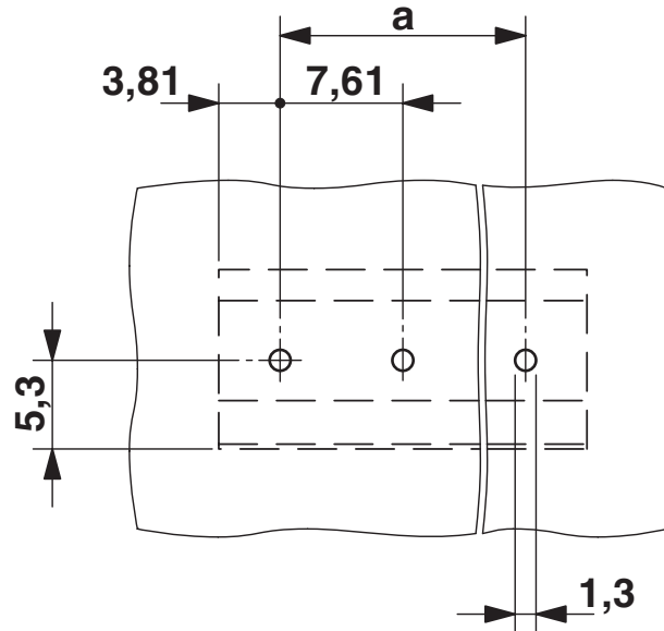
boorsjabloon/soldeerpadgeometrie
