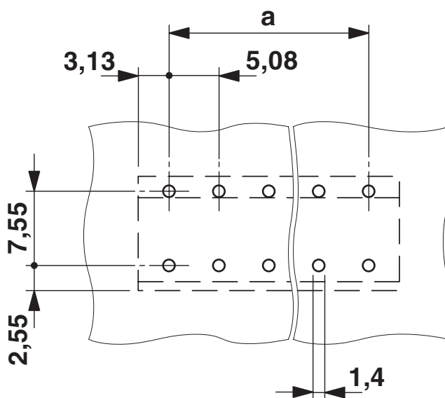
boorsjabloon/soldeerpadgeometrie
