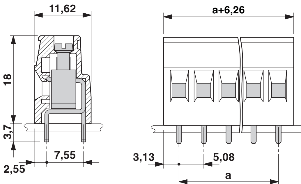
Maatschets
