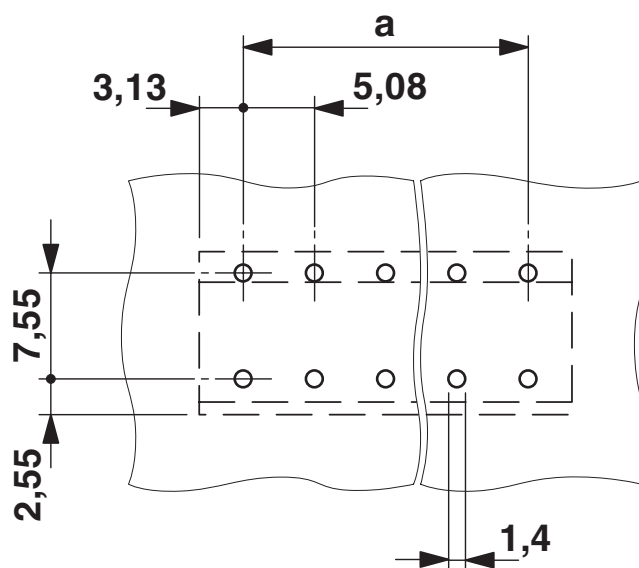
boorsjabloon/soldeerpadgeometrie
