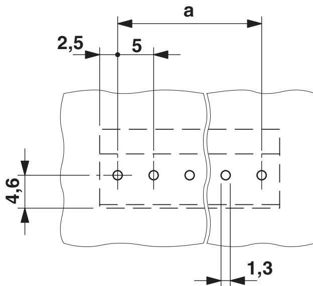
boorsjabloon/soldeerpadgeometrie
