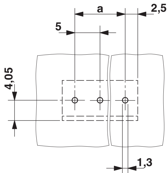
boorsjabloon/soldeerpadgeometrie
