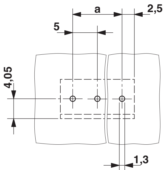
boorsjabloon/soldeerpadgeometrie
