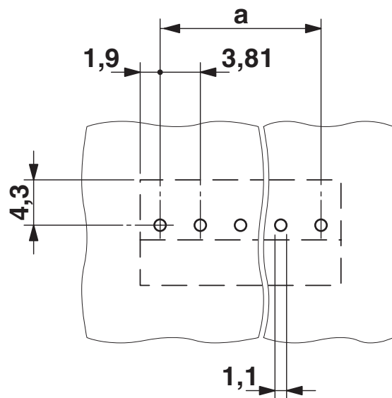
boorsjabloon/soldeerpadgeometrie
