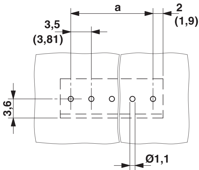
boorsjabloon/soldeerpadgeometrie
