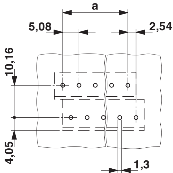
boorsjabloon/soldeerpadgeometrie
