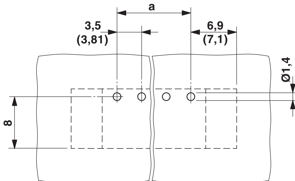
boorsjabloon/soldeerpadgeometrie
