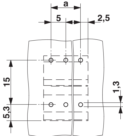
boorsjabloon/soldeerpadgeometrie
