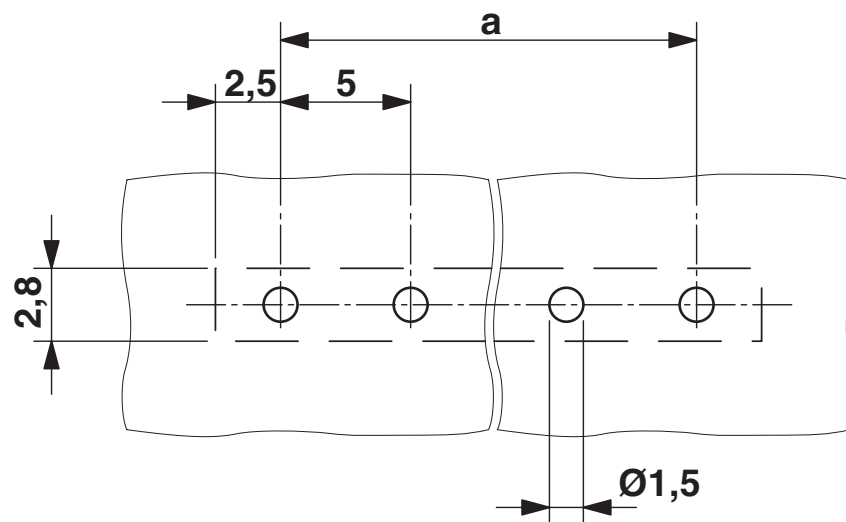
boorsjabloon/soldeerpadgeometrie
