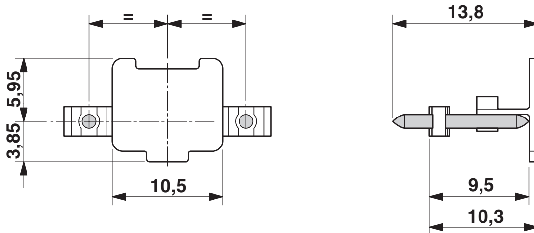
Maatschets
