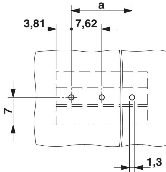
boorsjabloon/soldeerpadgeometrie
