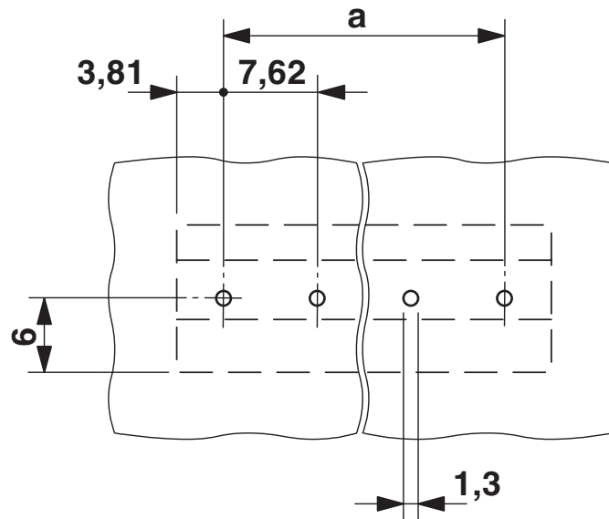
boorsjabloon/soldeerpadgeometrie
