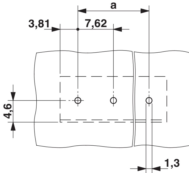
boorsjabloon/soldeerpadgeometrie
