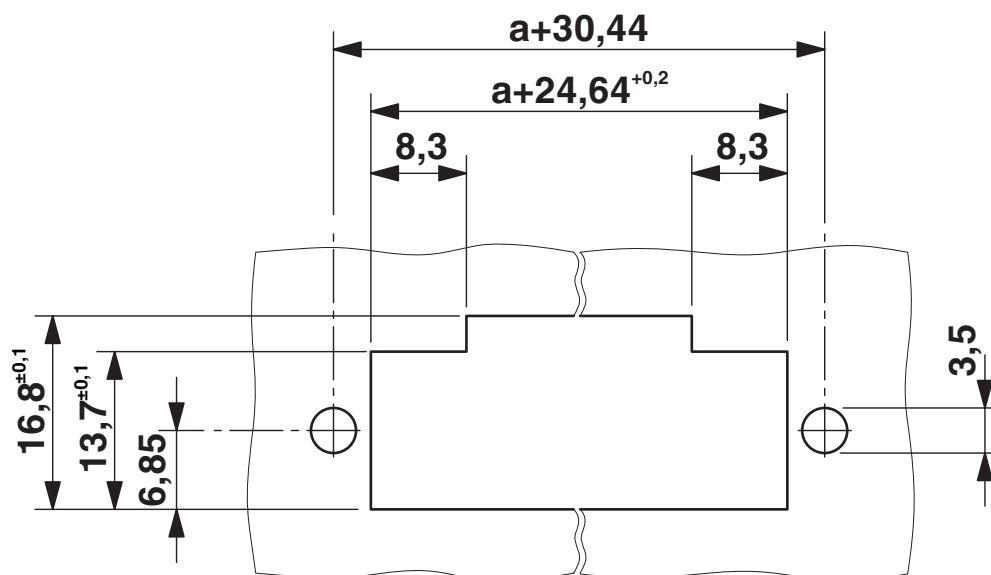
Uitsparing bij schroefbevestiging
