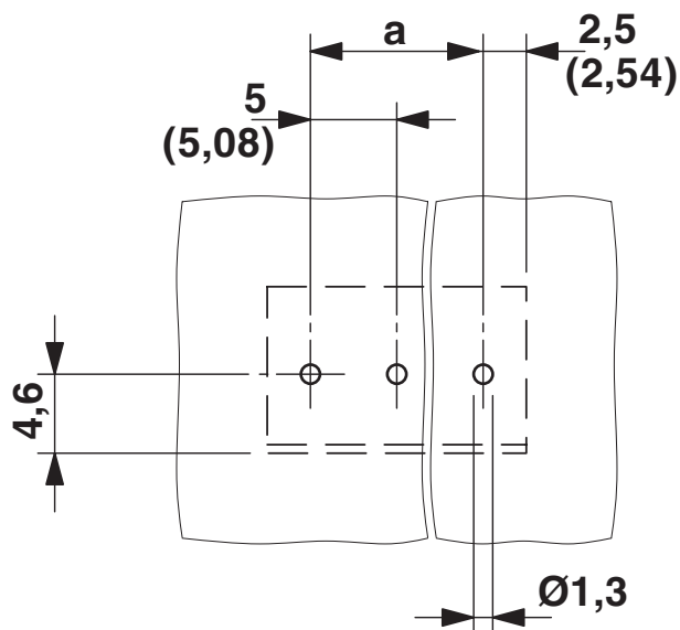
boorsjabloon/soldeerpadgeometrie
