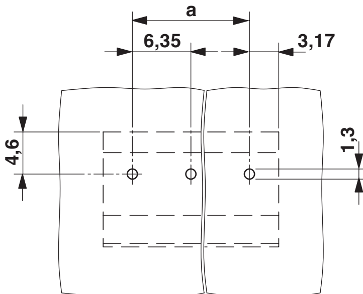
boorsjabloon/soldeerpadgeometrie
