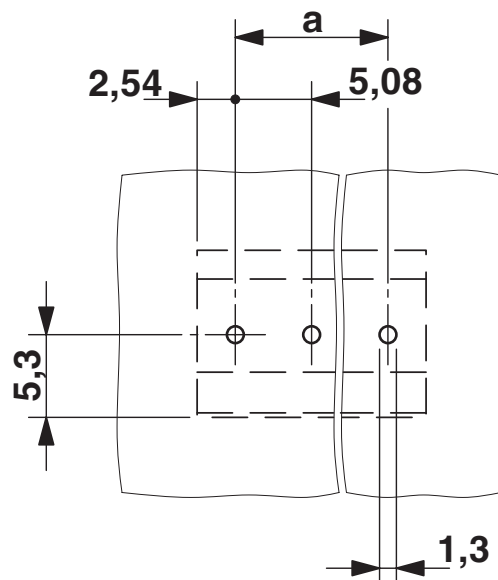
boorsjabloon/soldeerpadgeometrie
