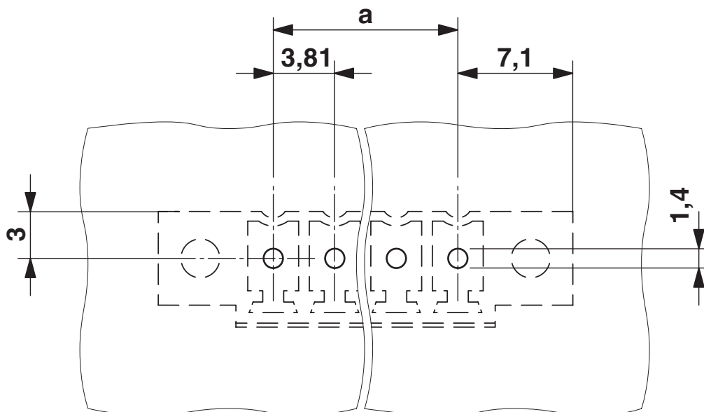
boorsjabloon/soldeerpadgeometrie
