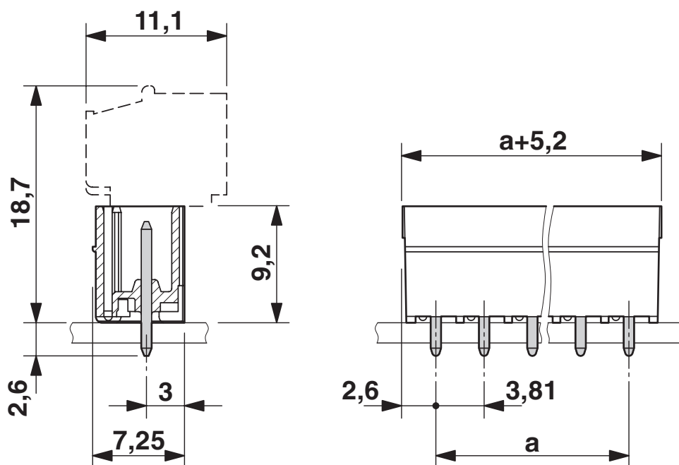
Maatschets
